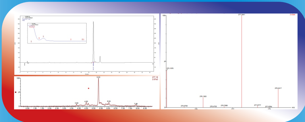
Kromatogram HPLC dan Profil MS Hasil Isolat 6-paradol
