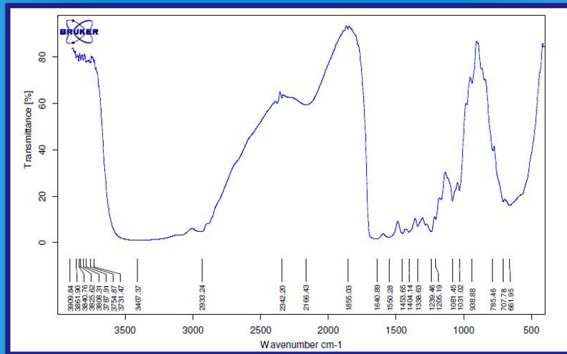
Spektrum IR Kalogen
